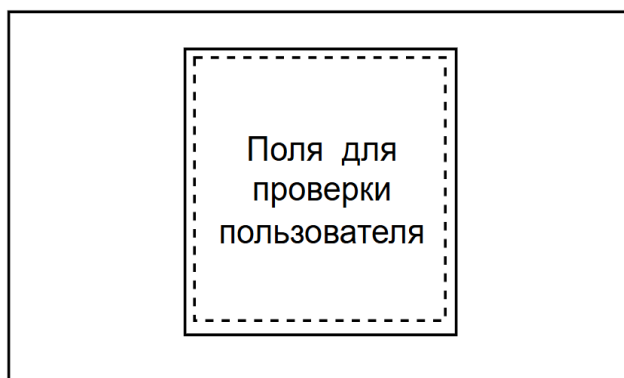
Рисунок 6. Макет profile.html
